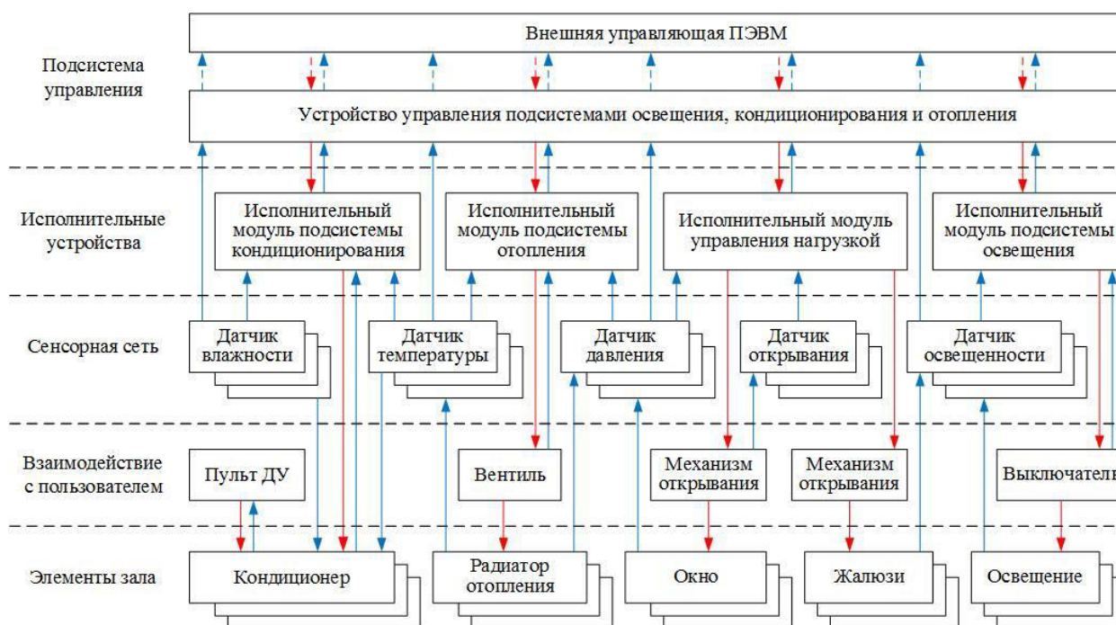
Рис. 2. Взаимосвязь подсистем жизнеобеспечения интеллектуального зала совещаний Fig. 2. Interconnection of the life support subsystems of meetings smart hall
